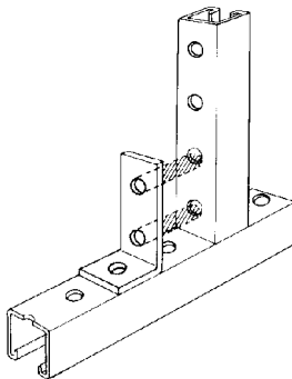
Kindorf 1 1/2"
